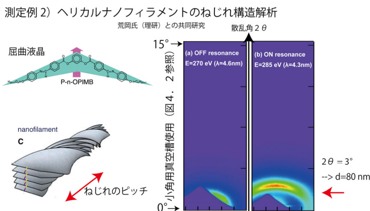
図 12-5-3: ヘリカルナノフィラメントのねじれ周期長の解析
